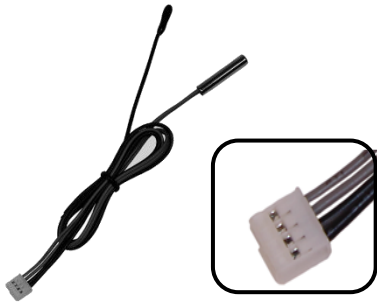
DSL LG SENSOR DUAL LG 10 \Omega AMB / 5 \Omega POZO
