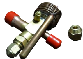
ETV22X-E VALVULA EXPANSIÓN 20TR IGUALADOR EXTERNO
